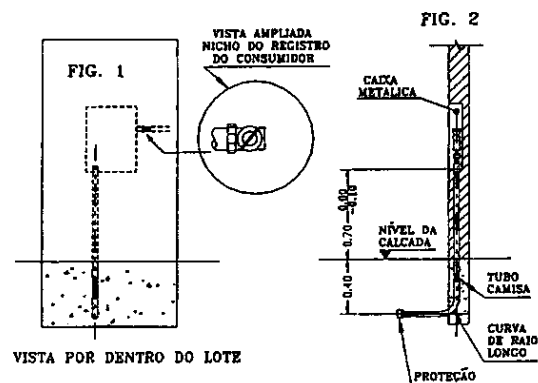
DETALHES PARA INSTALAÇÃO FRONTAL DA CAIXA DE PROTEÇÃO
