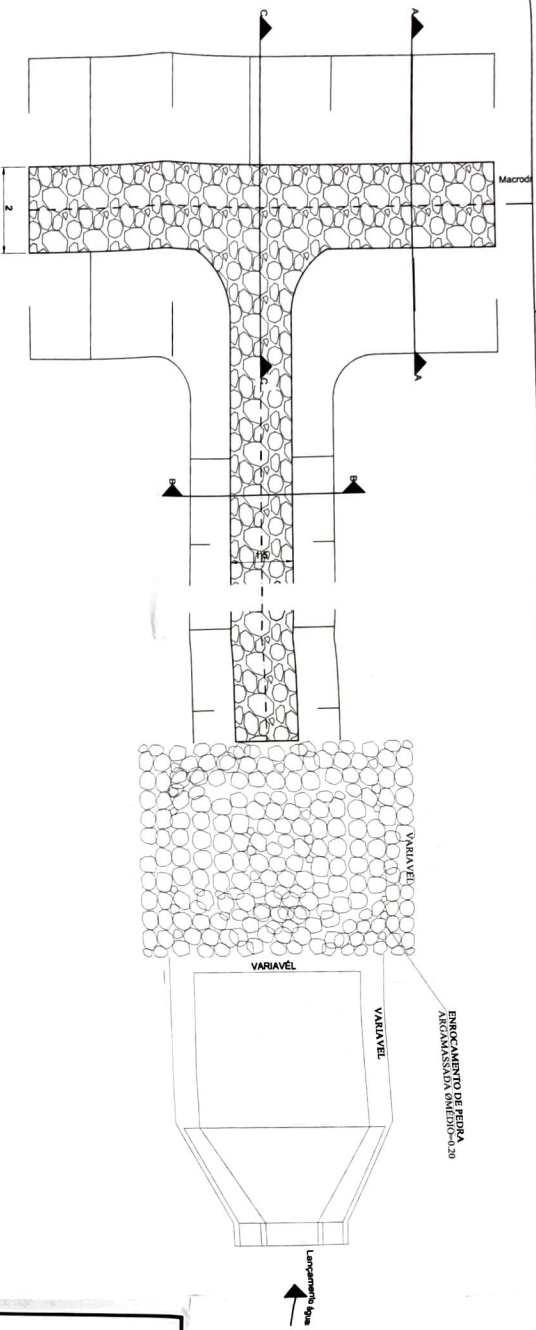
Planta de detalhe do canal de macrodrenagem com o lançamento de águas pluviais de rede projetada Escala 1:80
