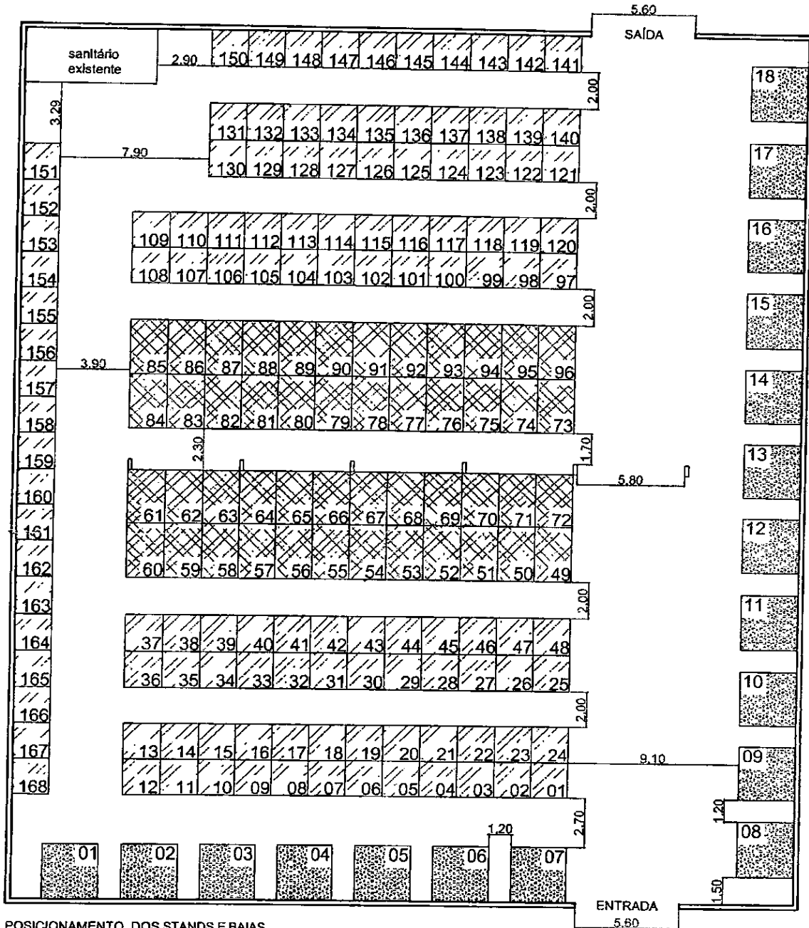
POSICIONAMENTO DOS STANDS E BAIAS escala 1:200
