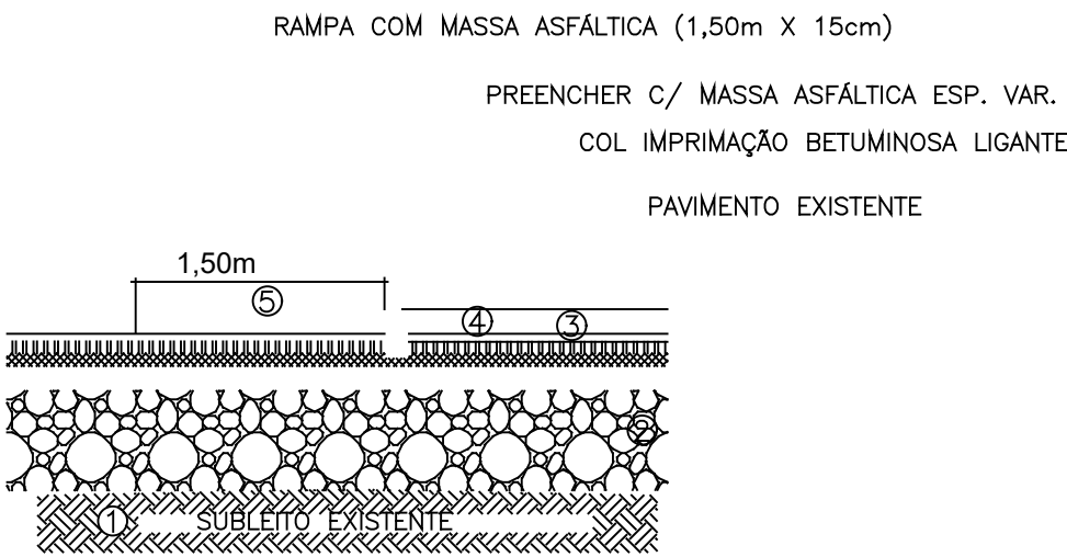
CORTE LONGITUDINAL
