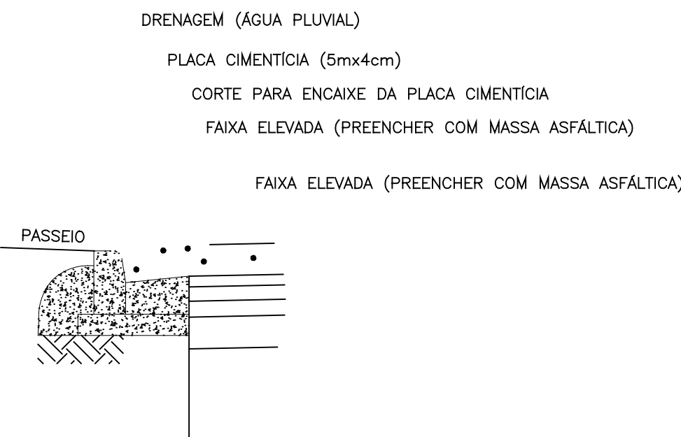
SEÇÃO-TIPO DA FAIXA ELEVADA S/ESC
