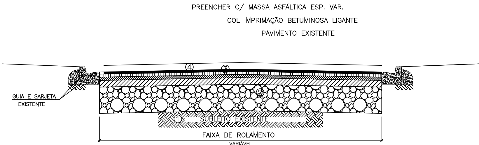
CORTE TRANSVERSAL
