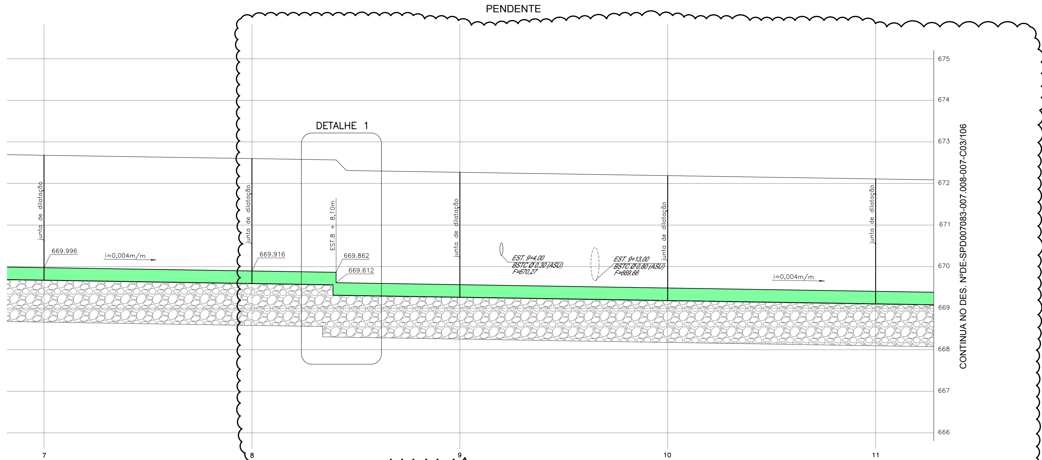
PERFIL LONGITUDINAL PELO EIXO DO CANAL ESC. VERT. 1:50 - HOR. 1:200
